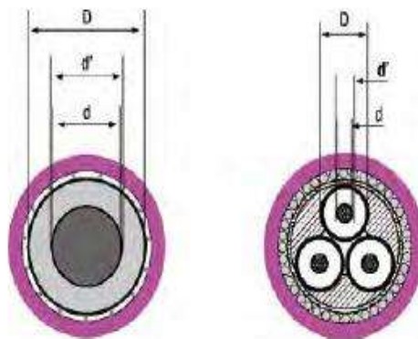
Figura 9. Diámetro de cuerda y semi interior del cable de la línea de evacuación
