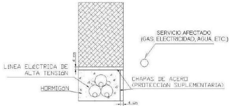
Figura 14. : Canalización de cables de energía
