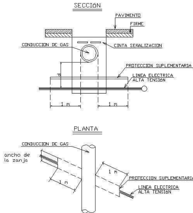
Figura 13. canalización de gas
