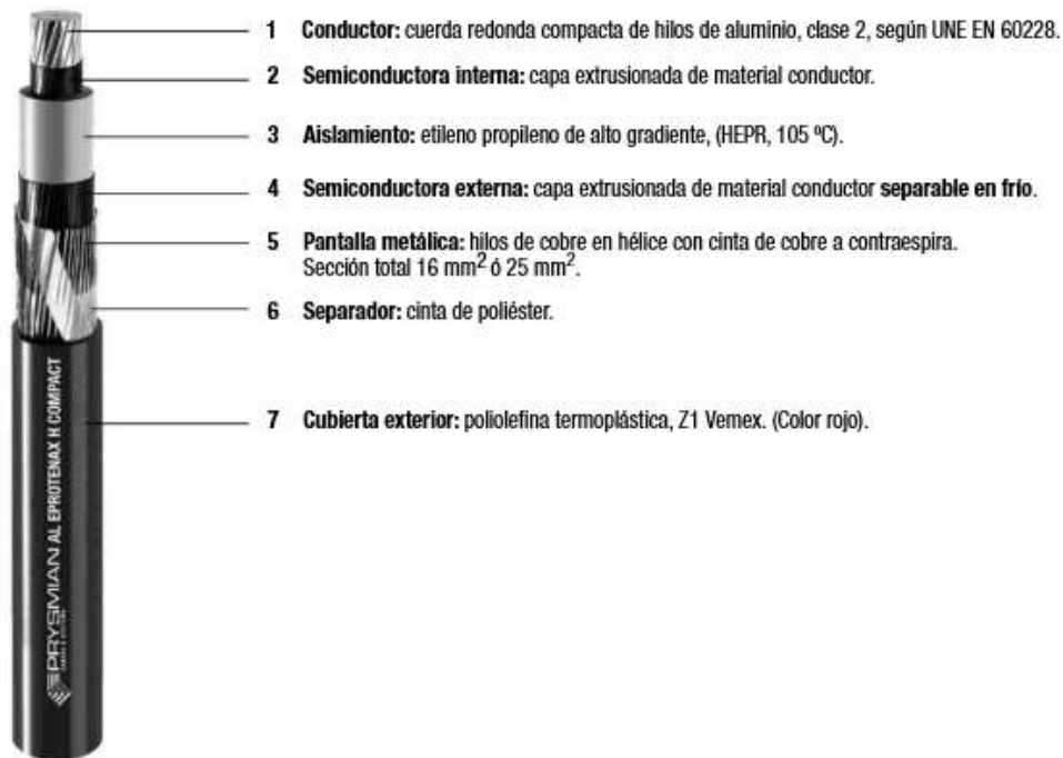
Figura 8. : Componentes de conductor de la línea de evacuación
