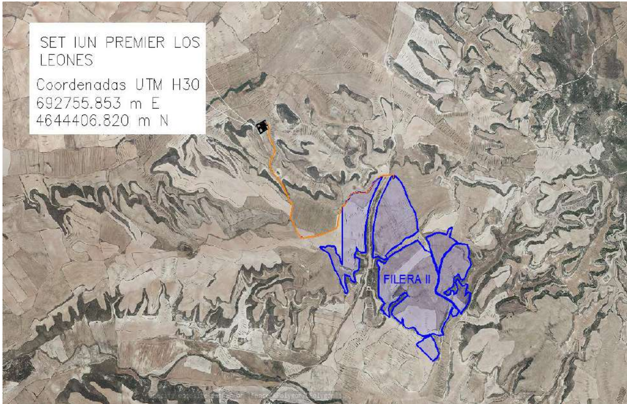
Figura 2. Ubicación de SE Filera II 30 kV y la Set Premier Los Leones30/220kV
