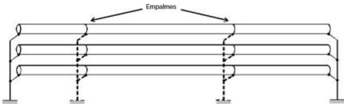
Figura 10. Esquema de conexión rígida a tierra
