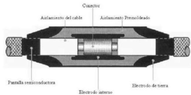
Figura 11. Figura de empalmes premoldeados
