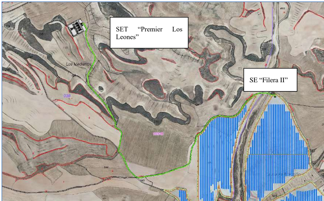
Figura 3. Trazado de la alternativa 1 subterránea. Fuente propia.
