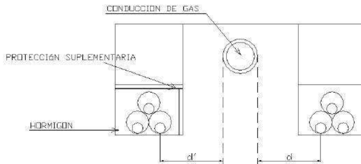
Figura 15. Canalización de cables de telecomunicación
